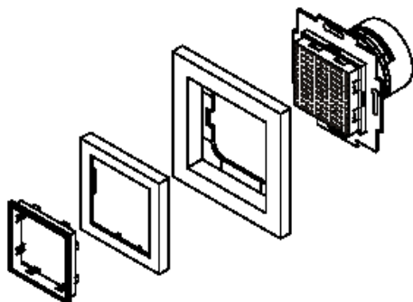
Obr. 2 – Sestavení přístroje s rámečkem a krytem
